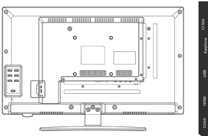
Geräte- Rückseite
